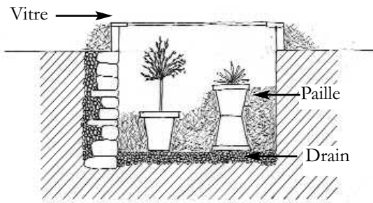
Fig 4 : la mini-serre enterrée
